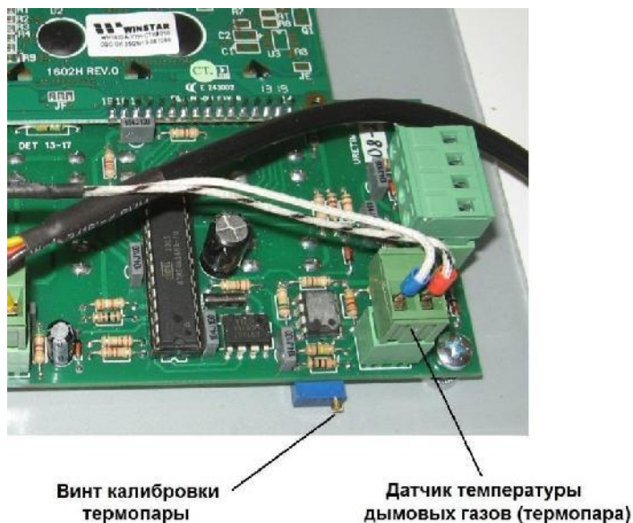
Рисунок 12. Калибровочный винт термопары.
